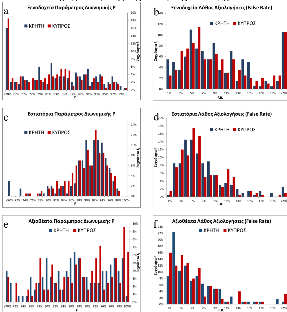
Εικόνα 4: Ιστογράμματα Προσέγγισης Διωνυμικής Κατανομής
