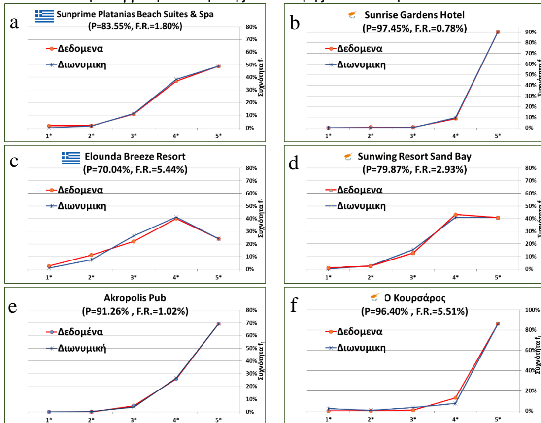
Εικόνα 3: Προσέγγιση Διωνυμικής Κατανομής στα Δεδομένα
